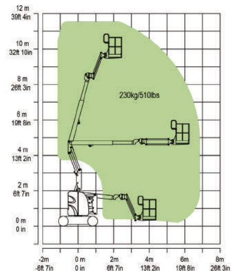
Bewegungsbereich ZA10RJE
